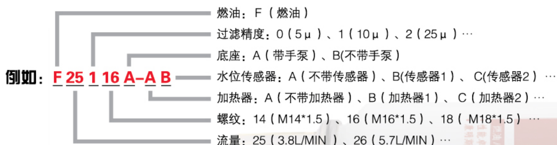
油水分离器编号规则以及说明
